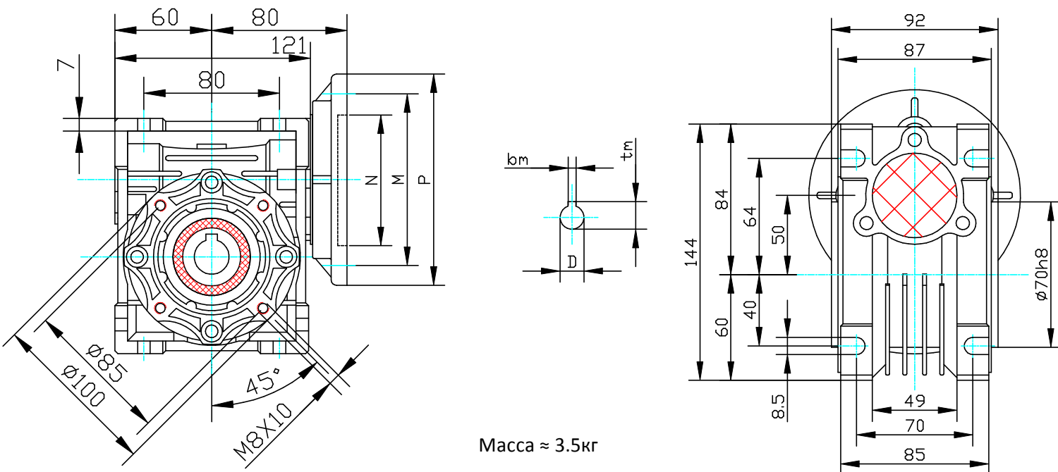
Выходной фланец.
