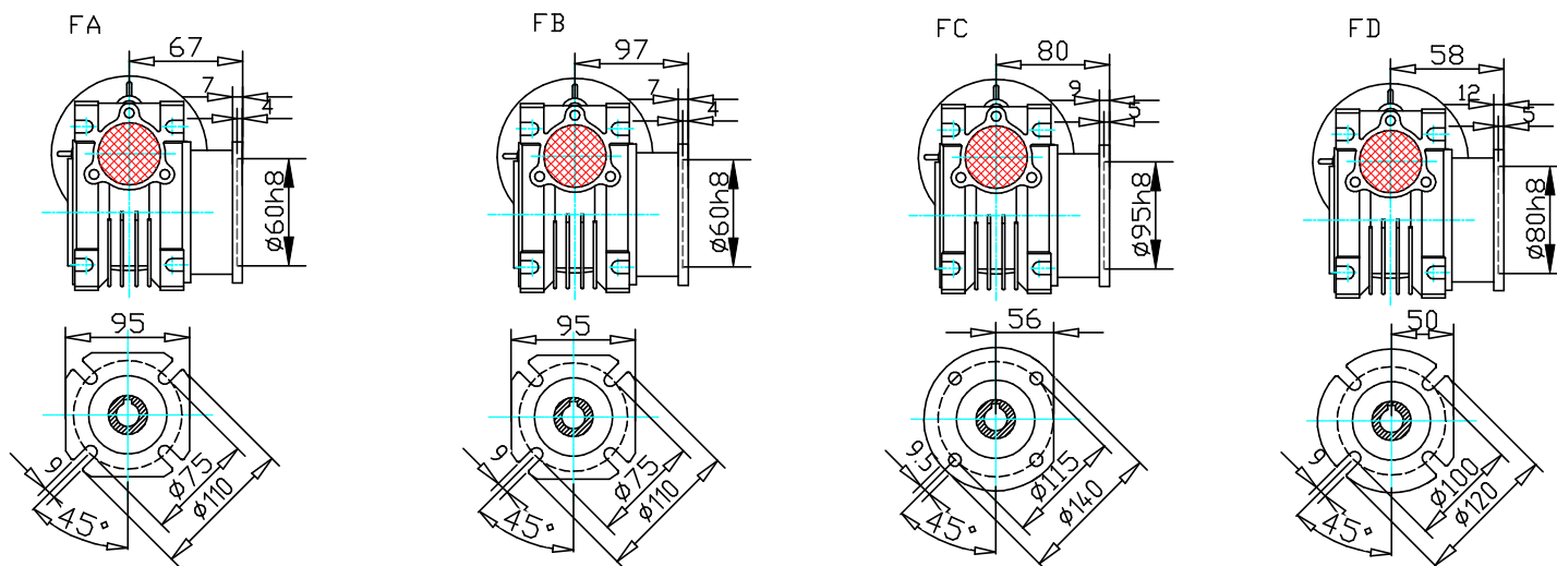
Выходной фланец.
