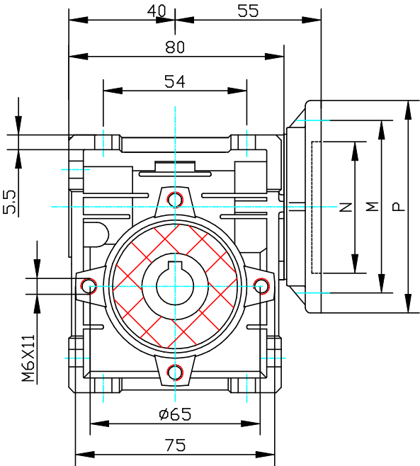
Выходной фланец.
