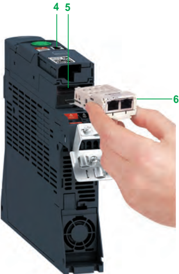
Пример установки коммуникационного модуля 6 (вид снизу) на преобразователь с блоком управления книжного исполнения
