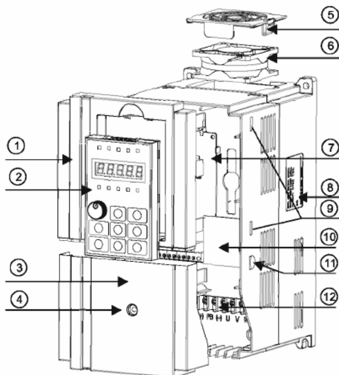
Рисунок 2-1 Принципиальная схема структуры преобразователя частоты
