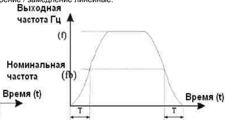
Рисунок 6-3 S-образная кривая разгона / торможения
