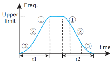
Рис.6-5 Разгон/замедление по кривой S
