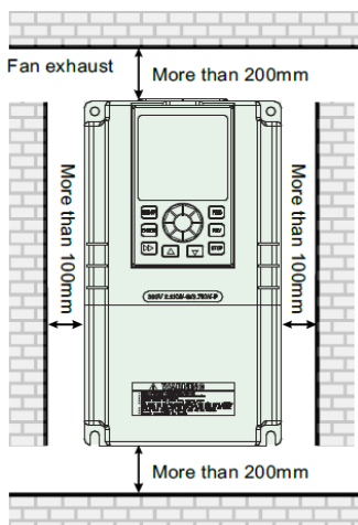
Рис.3-1. Монтажное пространство и расстояние
