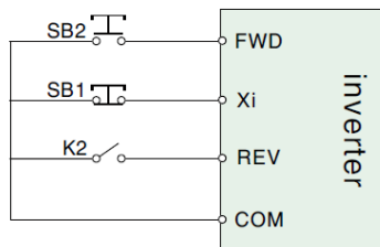
Рис.6-24 3-проводной режим управления 2
