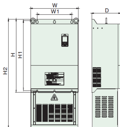
(b) Инверторы от 11кВт до 90кВт
