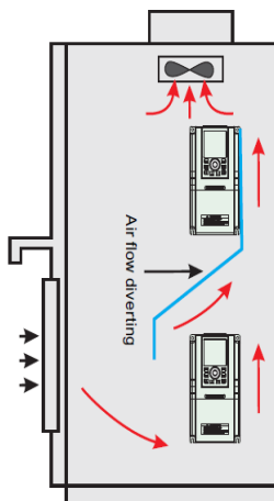
Рис.3-2 Монтаж нескольких инверторов
