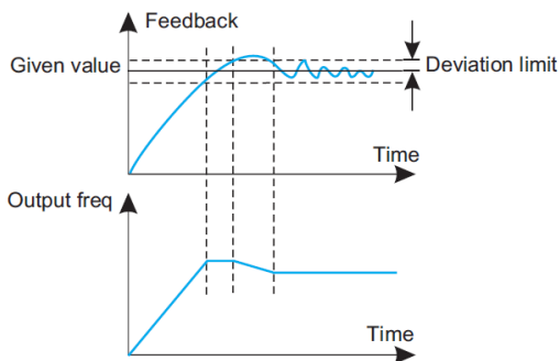
Рис.6-33 Предел отклонения
