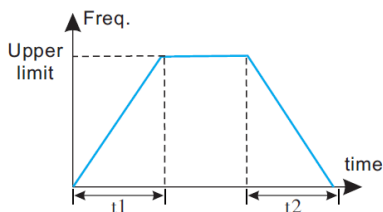
Рис.6-4 Линейный разгон/замедление
